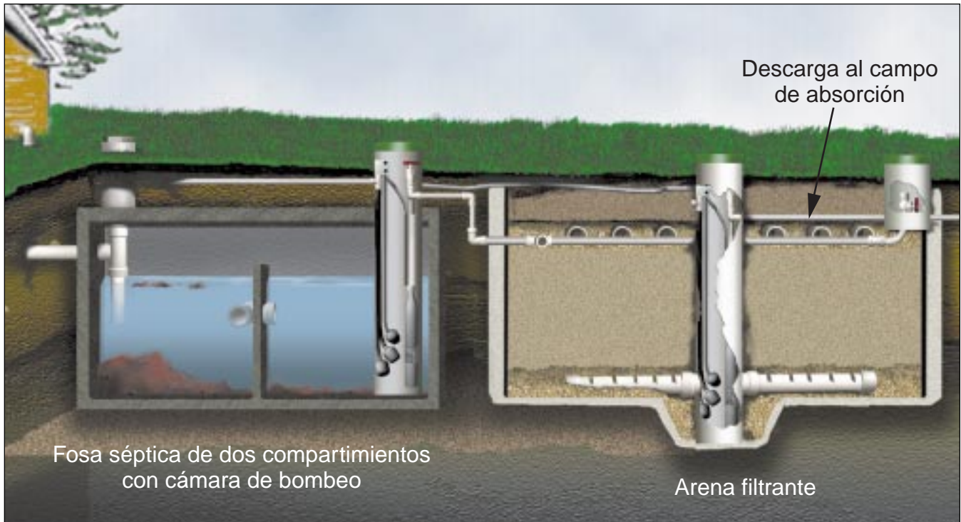
Figura 1: Un sistema de filtro de arena.
