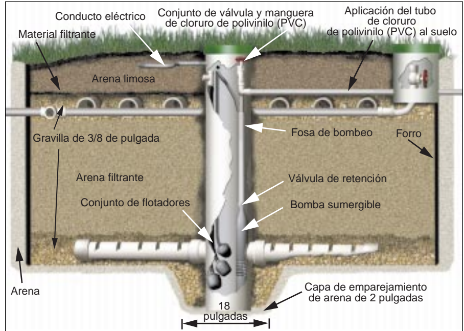
Figura 2: Un filtro de arena.
